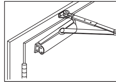
STANDARD MOUNT (PULL SIDE)
